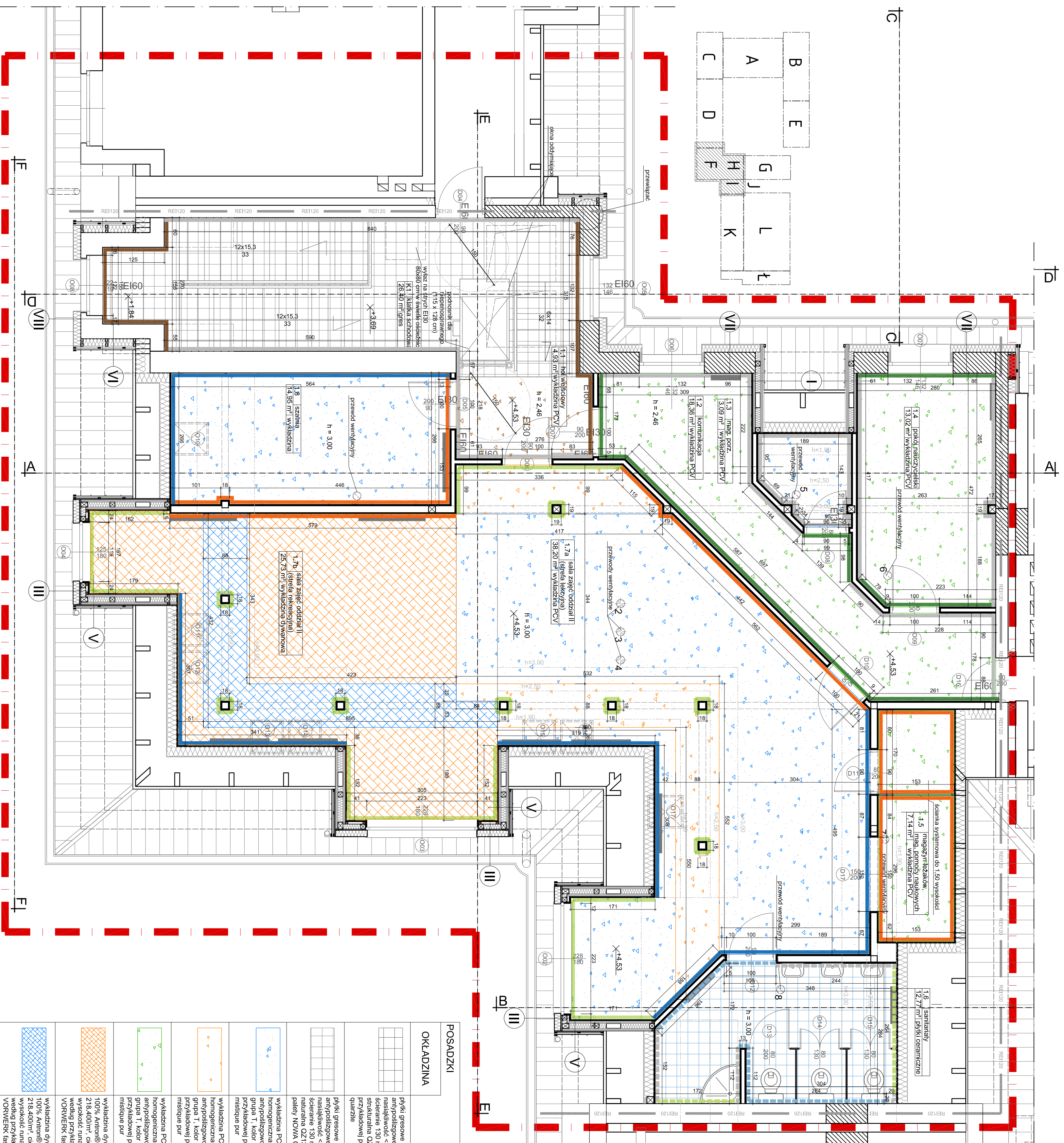
rzut poddasza
